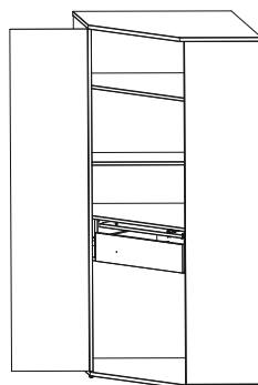
шкаф с дверями Т700/КУ 844x844x1858
